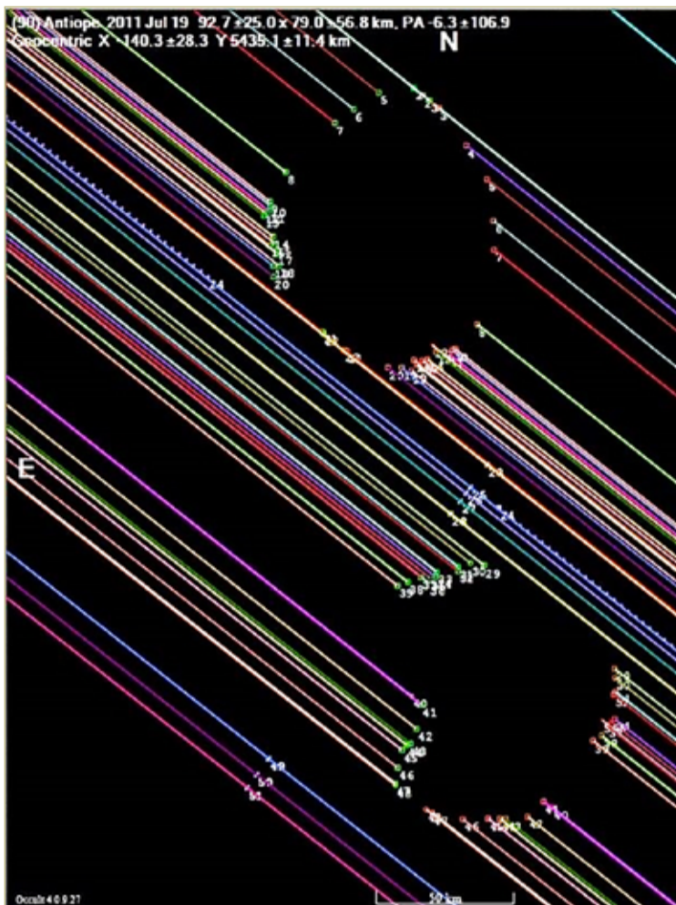
Сверху изображение двойного астероида Антиопа, построенное на данных одновременной съёмки 57 любительских телескопов в разных точках. Снизу то, как его видит 8-метровый телескоп VLT или Very Large Telescope — один из самых крупных на планете.
